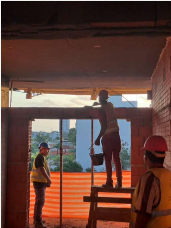
Trabajos de albañilería – Encofrado y armado de losa N8 – Fachada Torre Habitacional 1
