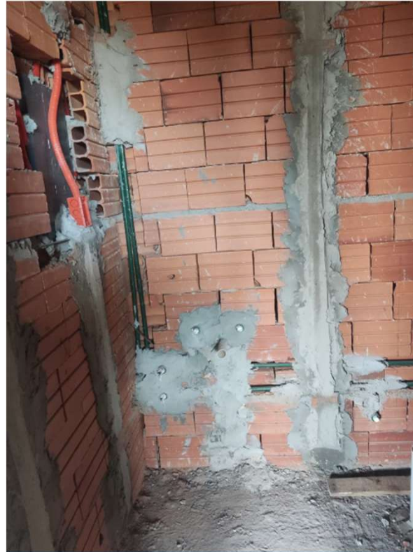
Trabajos de revoque en pasillos – Instalaciones de plomería – Trabajos de revoque e Instalaciones eléctricas
